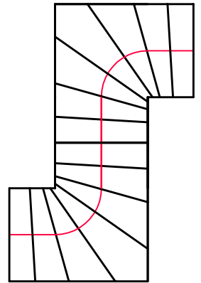
Type 5 - 2 Quarts Tournants Inversés
