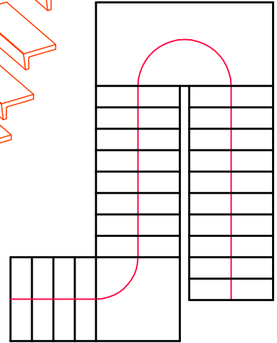
Volées Droites et Palier
