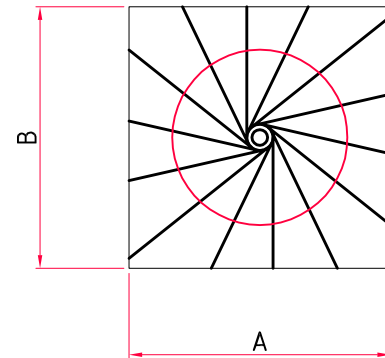
Marche de Départ
