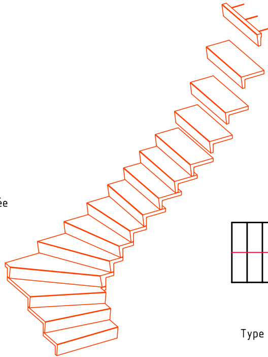
Type 4 - 2 Quarts Tournants avec Jour
