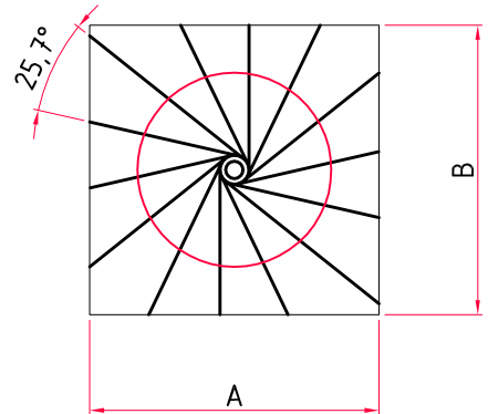
Marche de Départ
