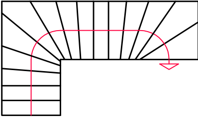
Type 2 - Quart Tournant et Arrivée Balancée
