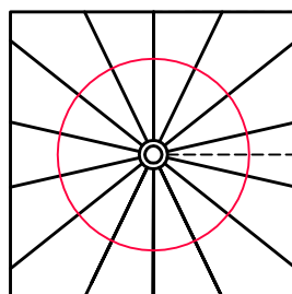
Hélicoïdal Trémie Carrée
